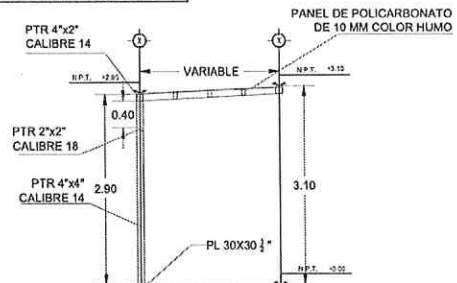
ALZADO LATERAL
