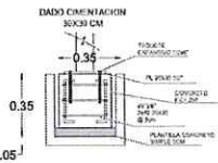
DETALLE DADO DE CIMENTACIÓN
