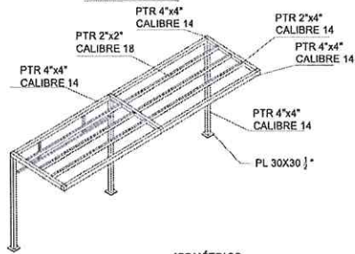
ISOMÉTRICO
